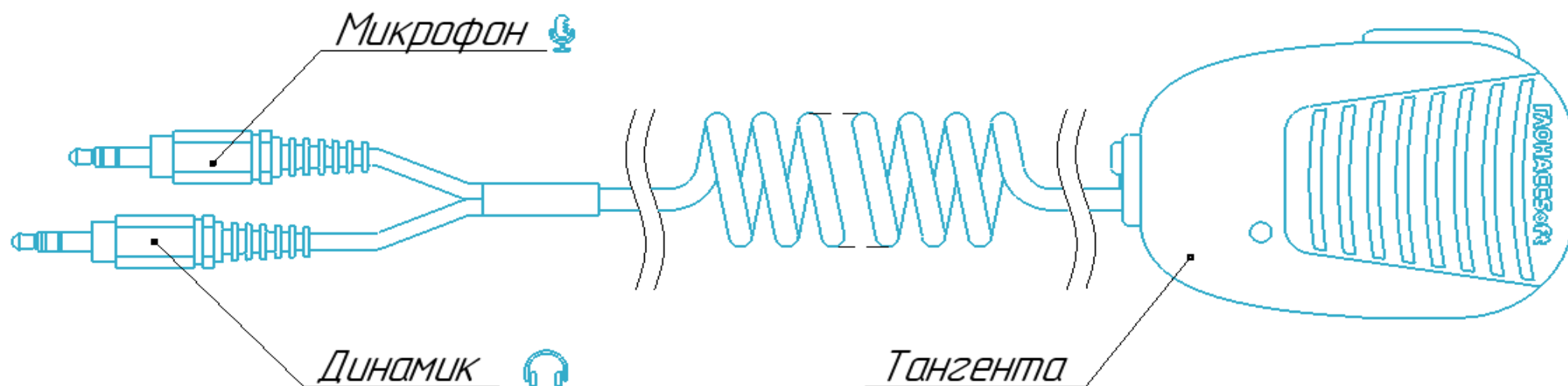
Рис 1: Тангента. Штекер динамика длинный провод. Штекер микрофона короткий провод.
